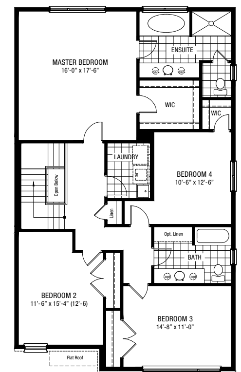
Elevation A
