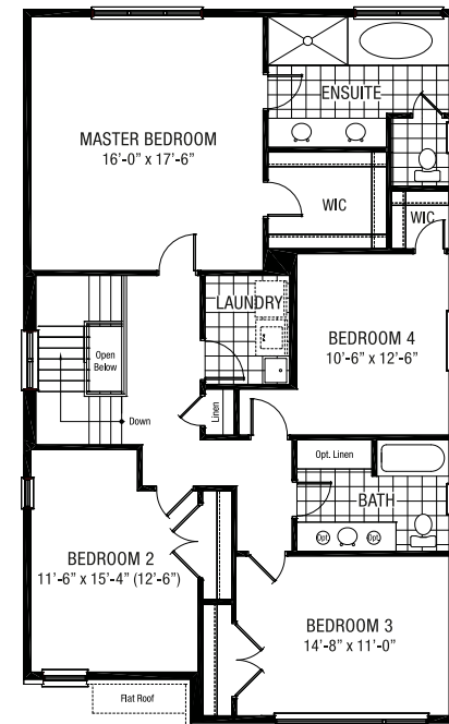
Elev. B
